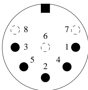
Abbildung 3: Funkgeräteanschluß
